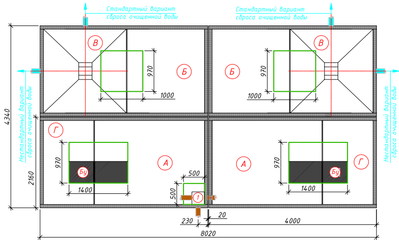
Схема станции
